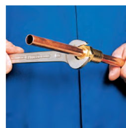
7. Apretar con una llave inglesa. 7. Apertar com uma chave inglesa.
